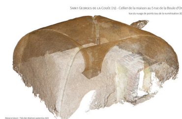
Cellier : vue du nuage de points issu de la numérisation 3D.
