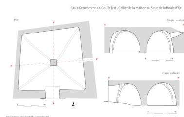
Cellier : plan et coupes.
