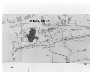
Projet définitif de construction de l'écluse, du barrage et du quai de l'impératrice : plan d'ensemble, vers 1860. Repro. François Lasa IVR52_20025300118X
