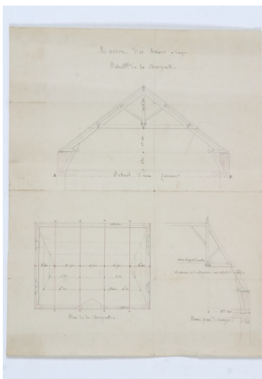
Projet de construction d'une maison pour les sœurs de Vaiges. Charpente : plan, ferme, demi-ferme de croupe, vers 1874. Repro. François Lasa IVR52_20045303219NUCA
