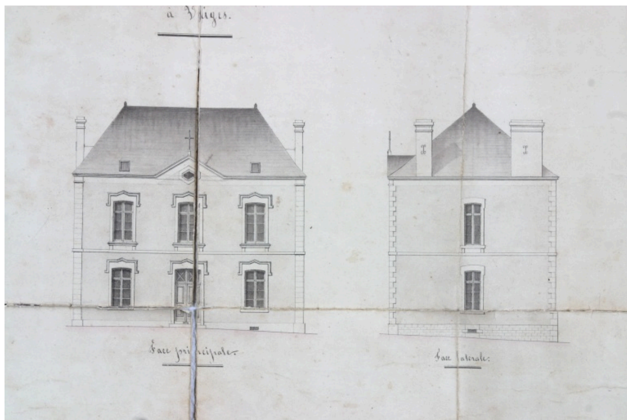
Projet de construction d'une maison pour les soeurs de charité de Vaiges (extrait) : élévation principale, élévation latérale, 1874.
