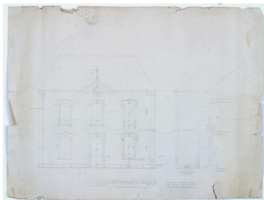
Projet de construction d'une maison pour les sœurs de Vaiges : élévation principale, élévation latérale partielle, coupe partielle, vers 1874. Repro. François Lasa IVR52_20045301916NUCA
