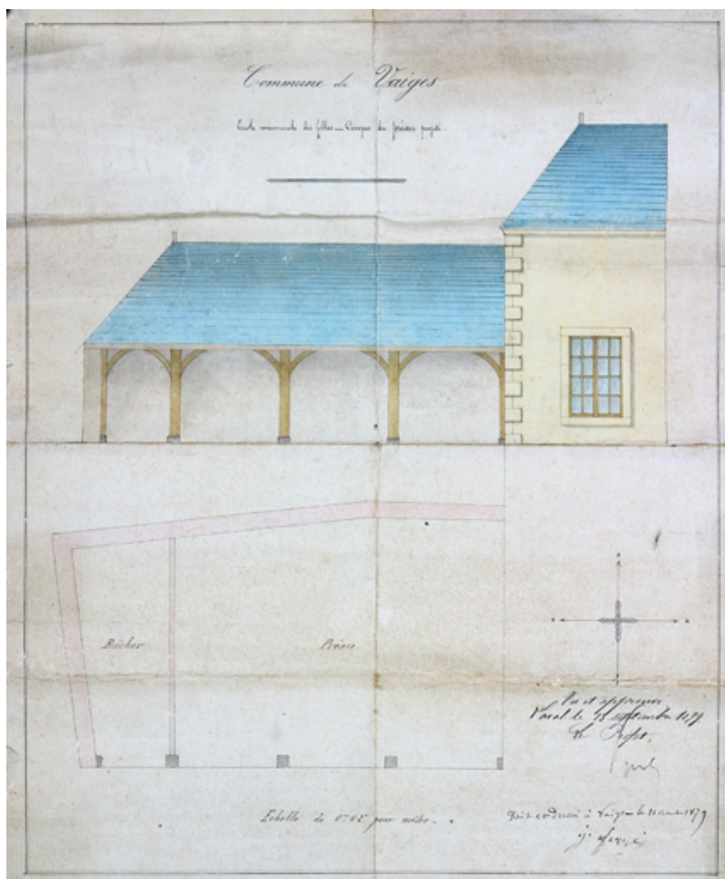
Projet de construction d'un préau et d'un bûcher pour l'école de filles : plan et élévation, 1879.
