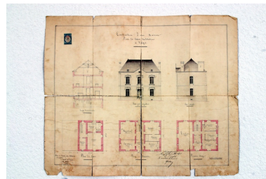
Projet de construction d'une maison pour les sœurs de charité de Vaiges : plans, élévation principale, élévation latérale, coupe transversale, 1874. Autr. Alexandre Dard, Repro. François Lasa IVR52_20045301421NUCA
