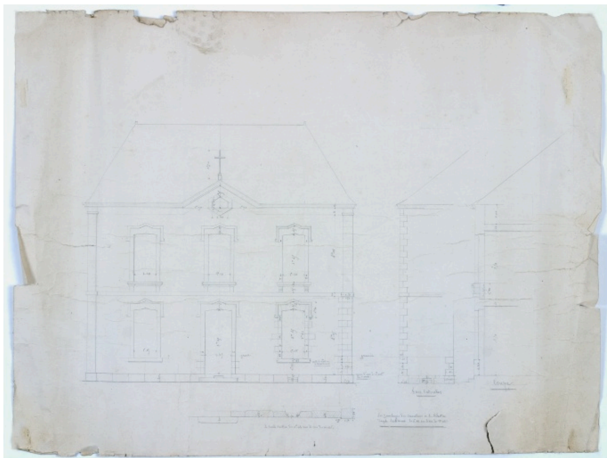
Projet de construction d'une maison pour les soeurs de Vaiges : élévation principale, élévation latérale partielle, coupe partielle, vers 1874.
