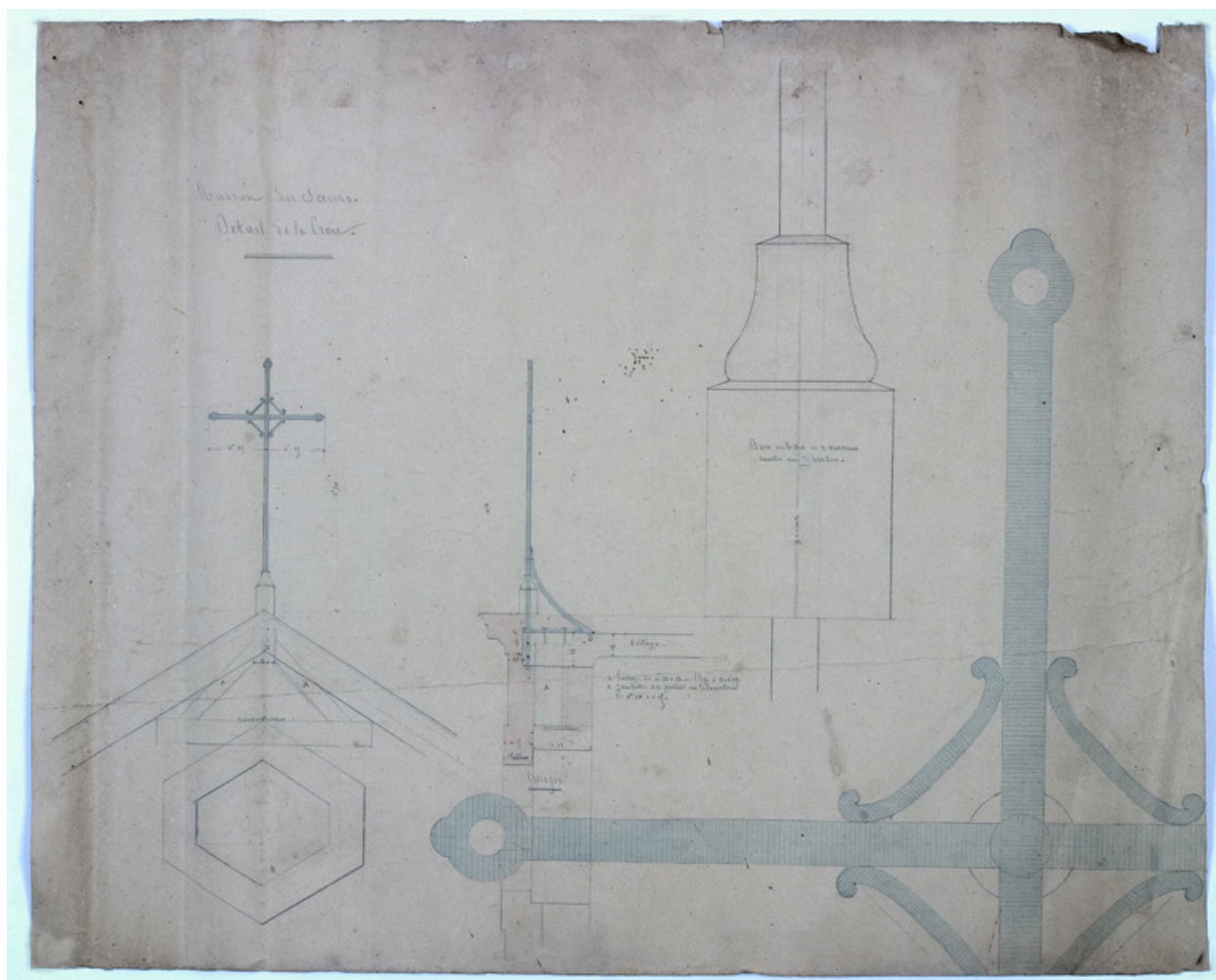
Projet de construction d'une maison pour les soeurs de Vaiges : détails de la croix, vers 1874.
