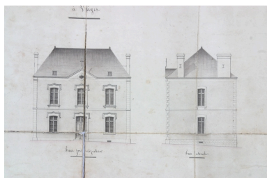
Projet de construction d'une maison pour les sœurs de charité de Vaiges (extrait) : élévation principale, élévation latérale, 1874. Autr. Alexandre Dard, Repro. François Lasa IVR52_20045301422NUCA
