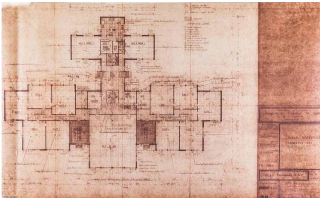
Plan de masse de l'école maternelle Sablon Est avec détail du revêtement de sols (Henri Wallon), 1980.
