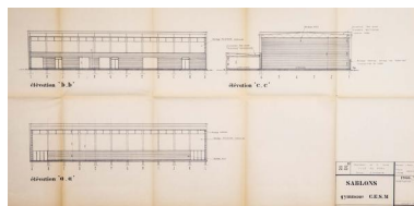
Elévation des façades pour le gymnase du collège Alain Fournier. Repro. Pierre-Bernard Fourny IVR52_20197200345NUCA
