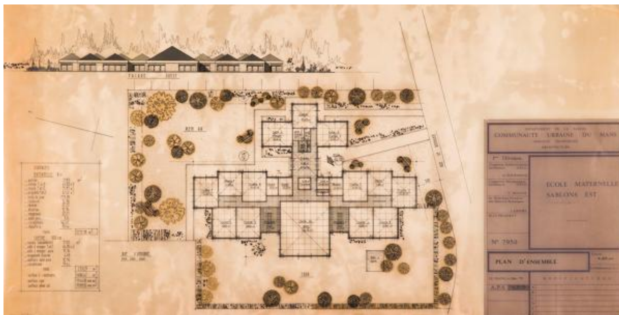
Plan d'ensemble et élévation de l'école maternelle Sablon Est (Henri Wallon) avec les plantations projetées, 1980.
