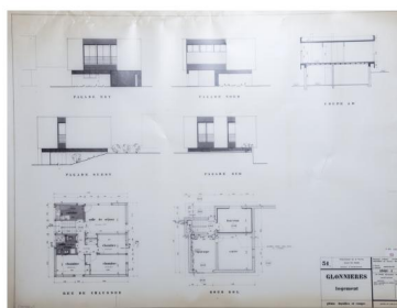
Elévation du logement de professeurs de l'école Guy Moquet aux Glonnières. Repro. Bruno Rousseau IVR52_20217200250NUCA
