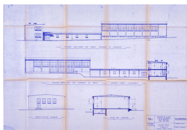
Vue des façades côté cour de l'école des Glonnières. Repro. Pierre-Bernard Fourny IVR52_20217200070NUCA
