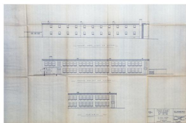
Elévation des façades de l'école Guy Moquet aux Glonnières. Repro. Bruno Rousseau IVR52_20217200258NUCA
