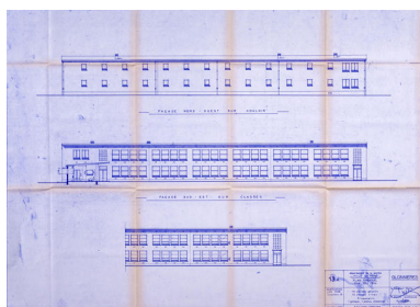
Elévation des façades sur rue de l'école des Glonnières. Repro. Pierre-Bernard Fourny IVR52_20217200069NUCA
