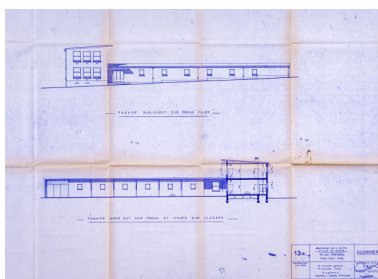
Vue des façades aile en retour de l'école des Glonnières. Repro. Pierre-Bernard Fourny IVR52_20217200073NUCA
