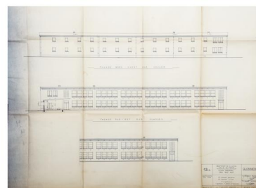
Elévation des façades de l'école Guy Moquet aux Glonnières. Repro. Bruno Rousseau IVR52_20217200257NUCA
