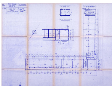
Plan du premier étage de l'école des Glonnières. Repro. Pierre-Bernard Fourny IVR52_20217200071NUCA
