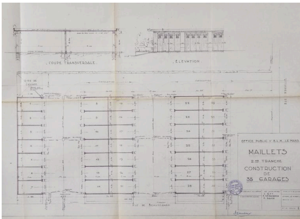
Plan, coupe et élévation des garages du groupe Brindenier, 1956.
