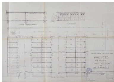
Plan, coupe et élévation des garages du groupe Brindenier, 1956. Repro. Pierre-Bernard Fourny IVR52_20197201705NUCA
