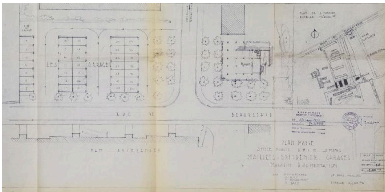
Plan-masse des garages et du magasin du groupe Brindenier, 1956.
