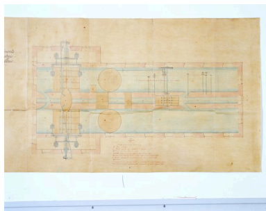
Plan du rez-de-chaussée de l'usine. Repro. François Lasa IVR52_20025300088XA
