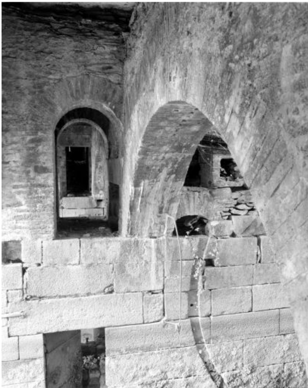
Vue de détail de la partie est du coursier latéral nord : mur bajoyer sud, arc, ouvertures donnant sur le coursier central, guide de la vanne qui épousait la forme de la roue.
