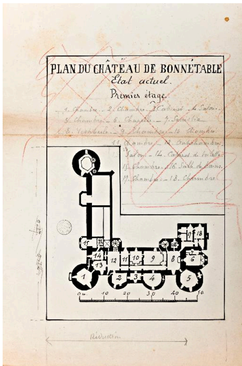
Plan du 1er étage du château en 1913
