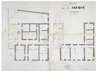
Plan du rez-de-chaussée et du premier étage (couleur grise) avant l'extension projetée en 1882 (couleur jaune). Autr. Louis Charpentier, Phot. Denis (reproduction) Pillet IVR52_20104400061NUCA
