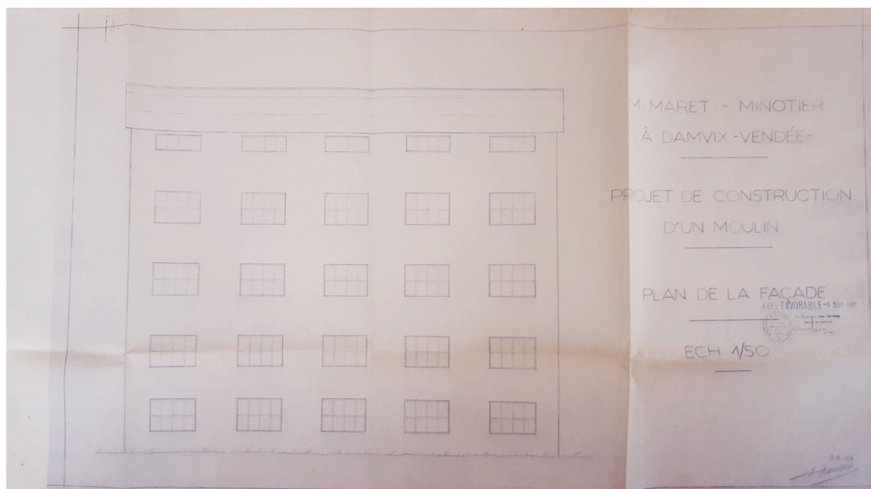
Projet de construction d'un bâtiment de broyage de la farine, 1963 : élévation sud.
