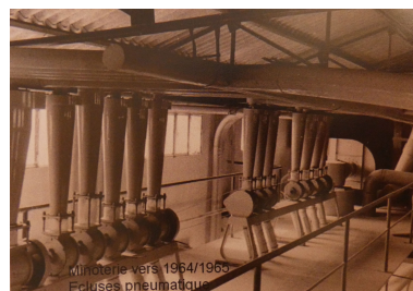
Ecluses pneumatiques dans la nouvelle minoterie vers 1964-1965. Phot. Yannis (reproduction) Suire IVR52_20228501344NUCA
