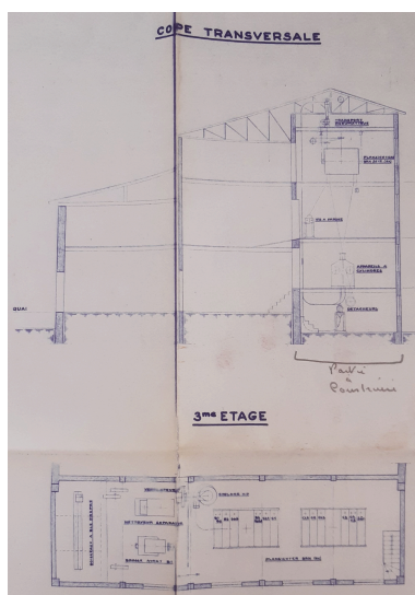
Projet de construction d'un bâtiment de broyage de la farine, 1963 : coupe transversale et plan du troisième étage. Phot. Yannis (reproduction) Suire IVR52_20228501068NUCA
