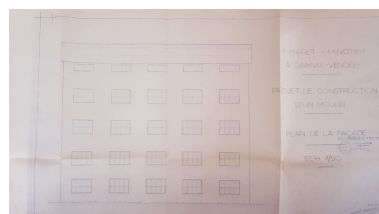
Projet de construction d'un bâtiment de broyage de la farine, 1963 : élévation sud. Phot. Yannis (reproduction) Suire IVR52_20228501066NUCA
