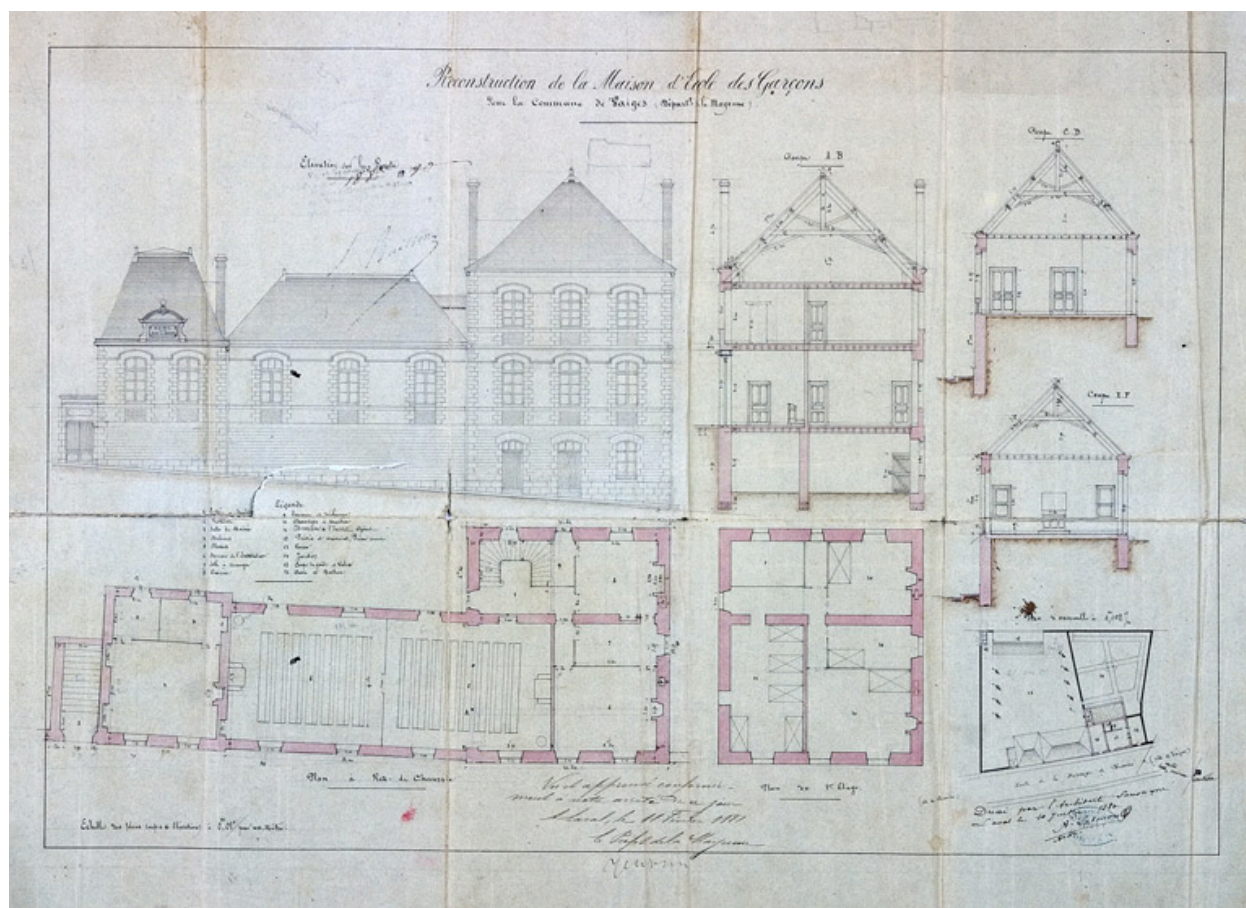
Projet de reconstruction de la mairie-école de garçons : plan-masse et de toiture, plan du rez-de-chaussée, plan de l'étage, élévation sur rue, coupes transversales, 1880
