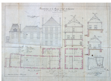
Projet de reconstruction de la mairie-école de garçons : plan- masse et de toiture, plan du rez-de- chaussée, plan de l'étage, élévation sur rue, coupes transversales, 1880 Autr. A. Salmon, Repro. François Lasa IVR52_20045301921NUCA
