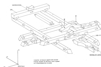
Moulin de Kercabus. Axonométrie de l'enrayure. 1972. Autr. Jean-Claude Delesne, Phot. Christian (reproduction) Cussonneau IVR52_20094401472NUCA
