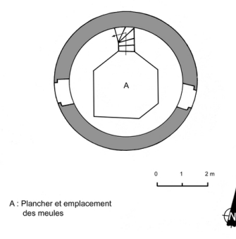
Moulin de Kercabus. Plan du 1er étage. Reprise de fond. 2009. Phot. Christian Cussonneau IVR52_20094401474NUCA
