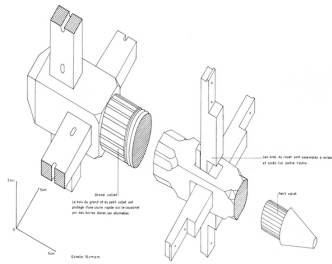
Moulin de Kercabus. Axonométrie de l'arbre tournant. 1972. Phot. Christian Cussonneau, Phot. Christian (reproduction) Cussonneau IVR52_20094401473NUCA
