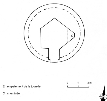
Moulin de Kercabus. Plan du rez- de-chaussée. Reprise de fond. 2009. Phot. Christian Cussonneau IVR52_20094401475NUCA
