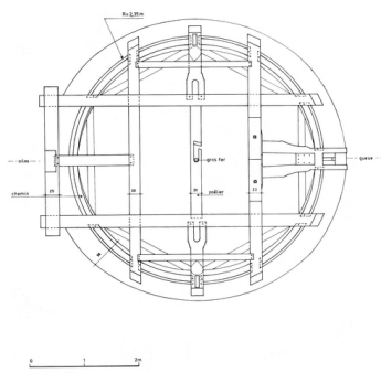
Moulin de Kercabus. Plan de l'enrayure. 1972. Autr. Jean-Claude Delesne, Phot. Christian (reproduction) Cussonneau IVR52_20094401471NUCA
