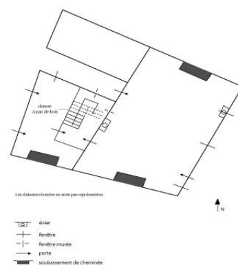
9 rue des capucins Plan schématique du rez-de-chaussée
