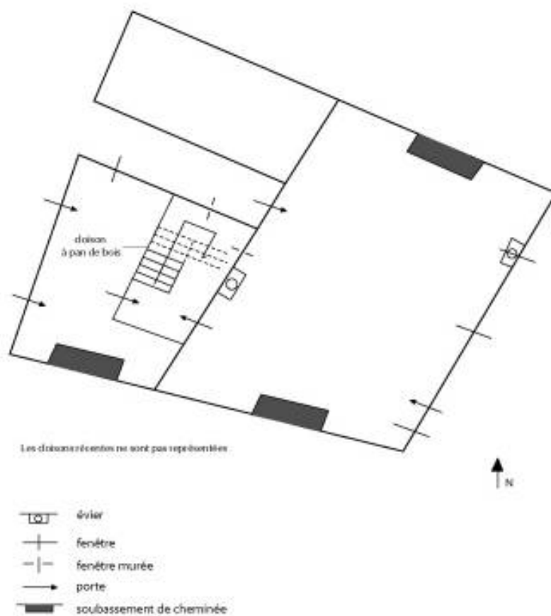
9 rue des capucins Plan schématique du rez-de-chaussée
