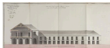
Coupe et élévation des façades projetées à l'ouest de la place du Marché, Mathurin Peccot, 3 mai 1813. Autr. Mathurin Peccot, Phot. Denis (reproduction) Pillet IVR52_20104400059NUCA
