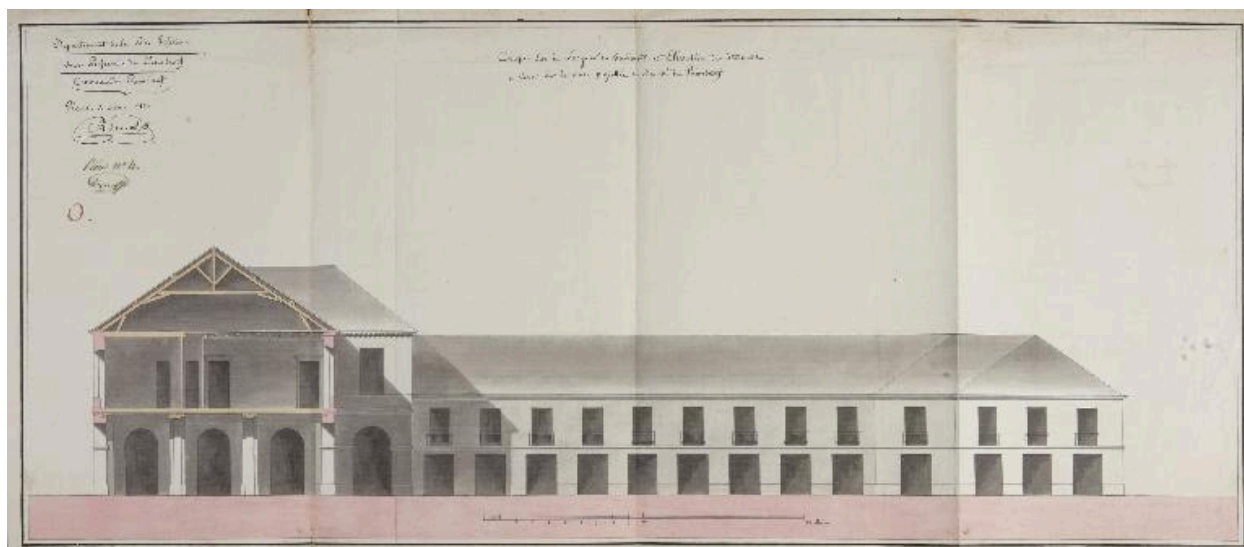
Coupe et élévation des façades projetées à l'ouest de la place du Marché, Mathurin Peccot, 3 mai 1813.
