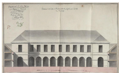
Élévation nord de l'ensemble à construire au sud de la place projetée, Mathurin Peccot, 3 mai 1813. Autr. Mathurin Peccot, Phot. Denis (reproduction) Pillet IVR52_20104400058NUCA
