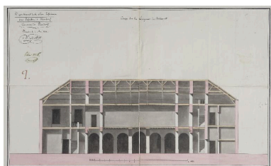
Coupe sur la longueur, Mathurin Peccot, 3 mai 1813. Autr. Mathurin Peccot, Phot. Denis (reproduction) Pillet IVR52_20104400060NUCA
