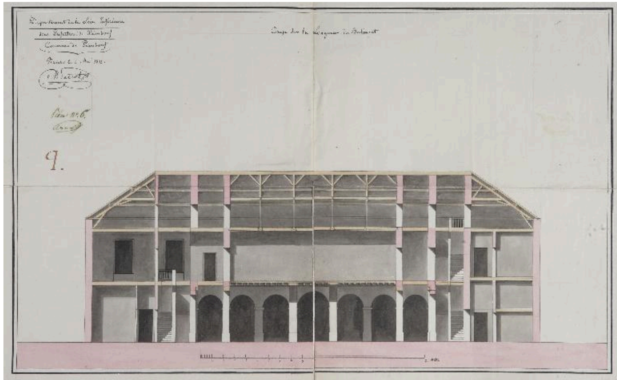
Coupe sur la longueur, Mathurin Peccot, 3 mai 1813.
