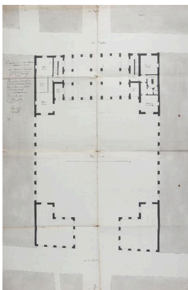
Plan du rez-de-chaussée de la halle à construire et de la place projetée, Mathurin Peccot, 3 mai 1813. Autr. Mathurin Peccot, Phot. Denis (reproduction) Pillet IVR52_20104400056NUCA
