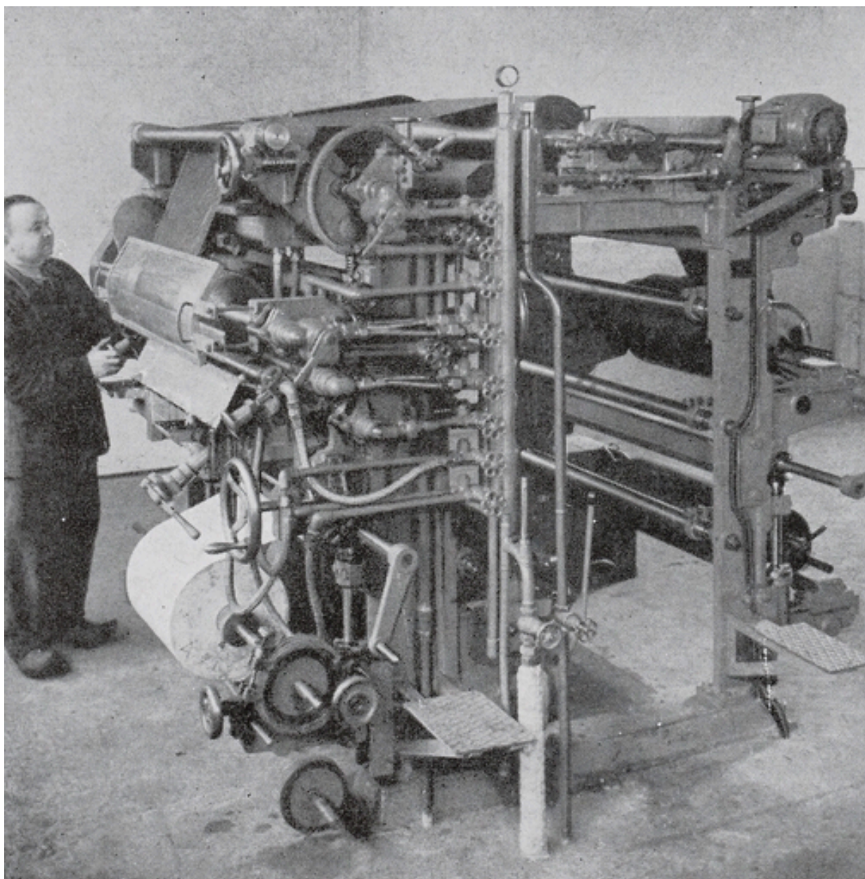
Machine à encrer les papier carbone, 1951.
