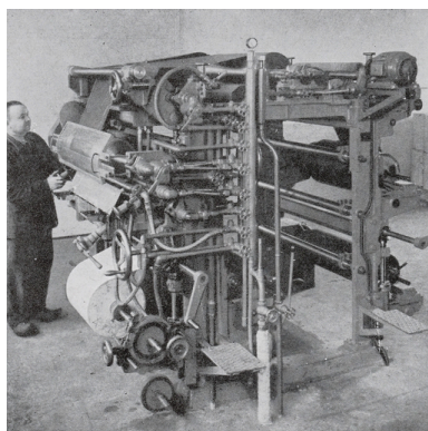
Machine à encre les papier carbone, 1951. Phot. Denis (reproduction) Pillet IVR52_20104400814NUCA
