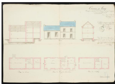
Projet de construction de l'école de garçons, Saint-Fraimbault, 1886. Repro. Morgane Acou-Le Noan IVR52_20205300549NUCA
