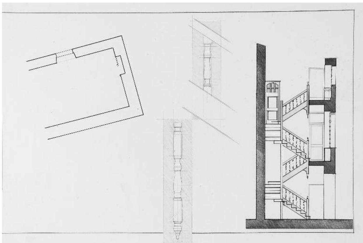
Coupe de l'escalier avec détails de ballustres.
