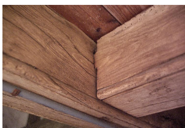
Le corps en appentis situé au sud, détail des solives. Phot. Denis Pillet IVR52_20034400481NUCA
