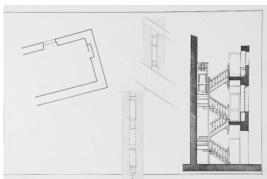
Coupe de l'escalier avec détails de ballustres. Autr. Jocelyn Bourneuf, Phot. Denis (reproduction) Pillet IVR52_20034401953NUC
