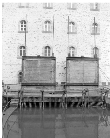
Vue de face des vannes motrices situées sur le flanc nord de l'ancien moulin.
