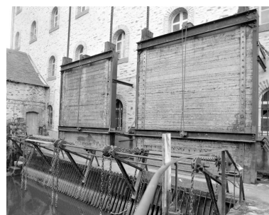
Les vannes motrices situées sur le flanc nord du moulin.
