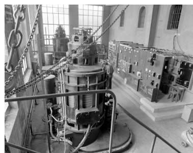
La salle des machines. Vue d'ensemble depuis la galerie est : à gauche, machine énergétique ; à droite, tableau de commande. Phot. François Lasa IVR52_20015300513X
