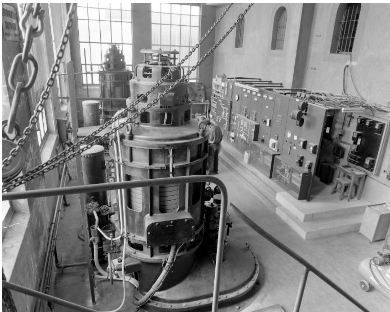
La salle des machines. Vue d'ensemble depuis la galerie est : à gauche, machine énergétique ; à droite, tableau de commande.
