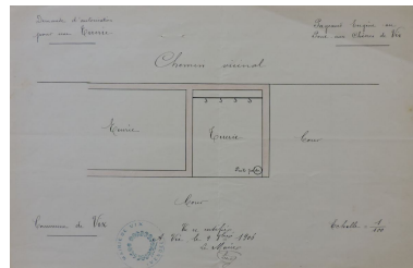
Plan de la tuerie établie dans le prolongement du bâtiment le long de la rue, 9 octobre 1906. Phot. Yannis (reproduction) Suire IVR52_20198503647NUCA
