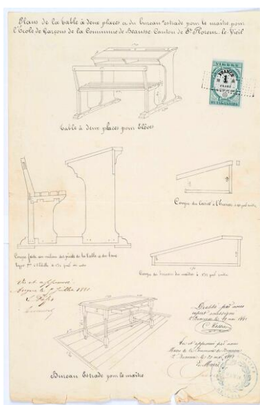
Plans d'une table à deux places et du bureau estrade pour le maître pour l'école de garçons de la commune de Beausse. Dressés par Tessier, menuisier, à Beausse, le 19 mai 1881. (AM Beausse ; 1 M 15). Repro. Armelle Maugin IVR52_20244901092NUCA
