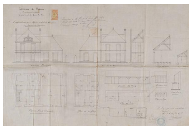
Projet de construction d'une maison d'école de garçons. Dressé par Anatole Bréheret, architecte, le 10 juin 1879. (AM Beausse ; 1 M 15). Repro. Armelle Maugin IVR52_20244901124NUCA
