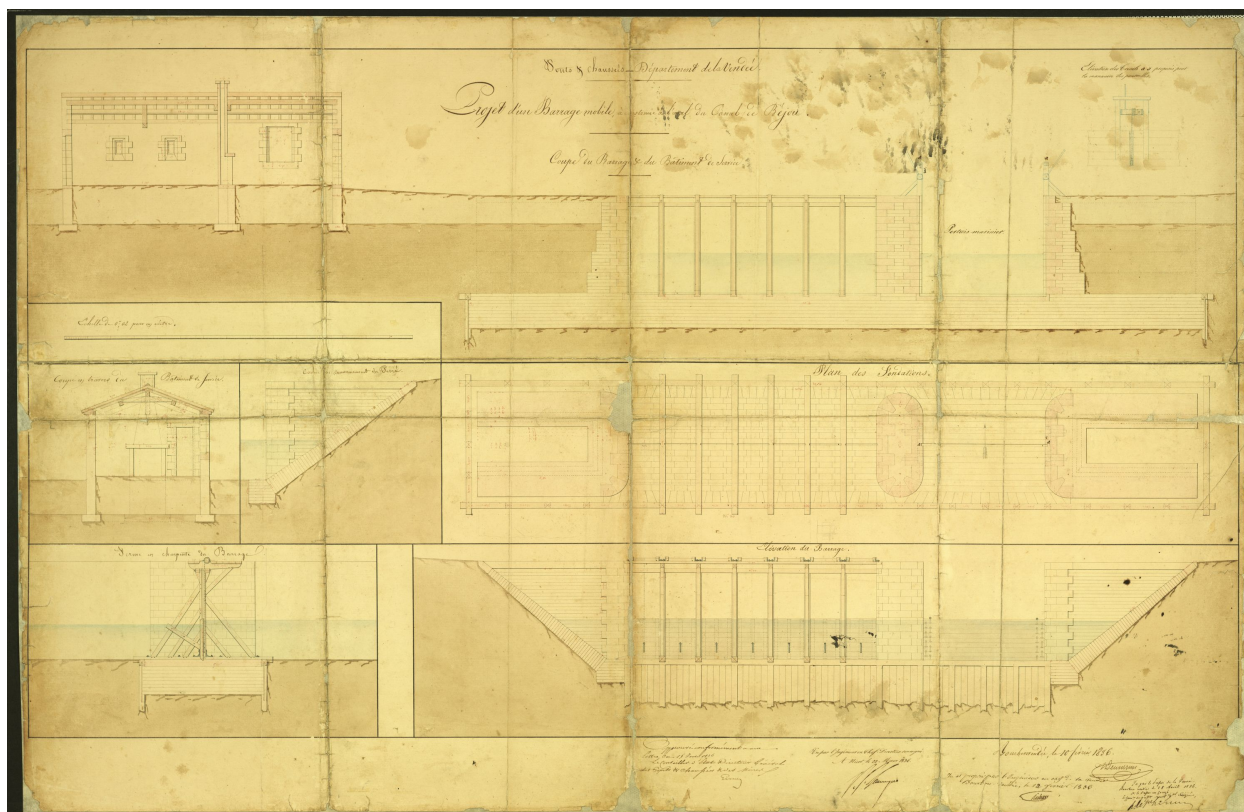
Projet de maison éclésièrre et de barrage pour le canal du Nouveau Bézou, 10 février 1836.
