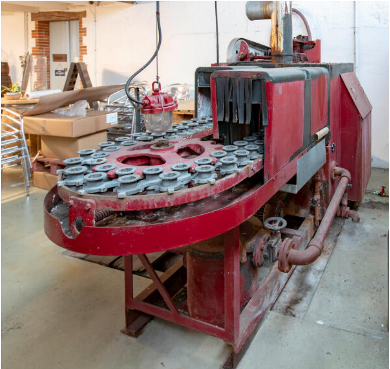
Laveuse à bouteilles dite "Girondine".
