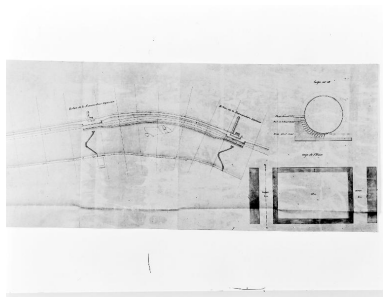
Projet de construction d'un moulin à Rochefort : plan des deux barrages de la Fourmondière supérieure et de la Fourmondière inférieure, plan au sol du moulin et coupe de l'une des roues.
