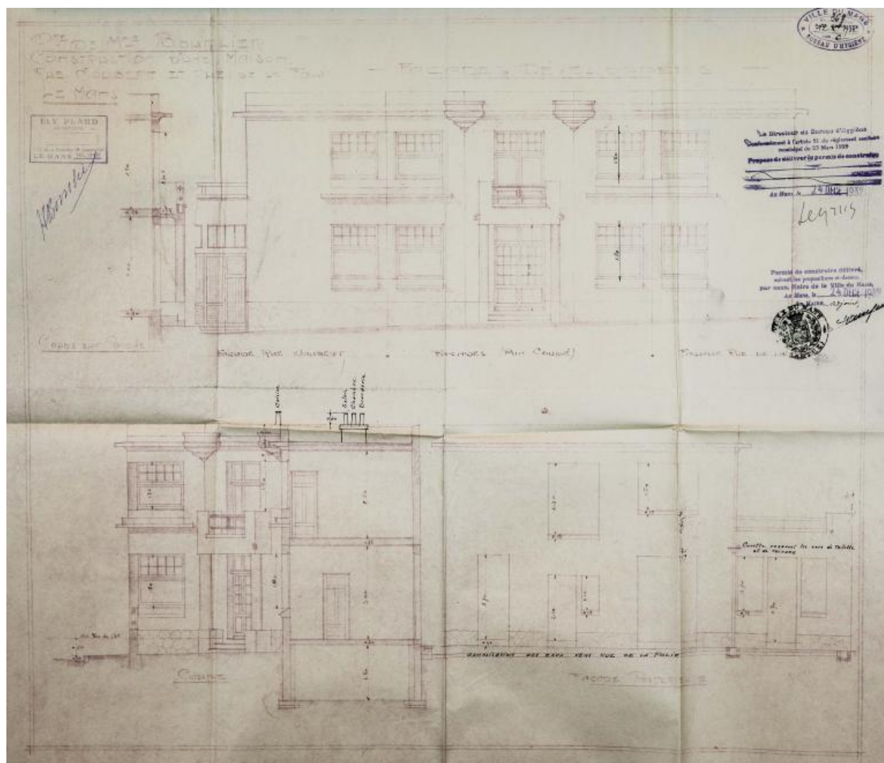
Elévation et coupe de la maison signées Ely Plard, 1934.
