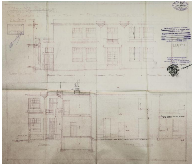
Elévation et coupe de la maison signées Ely Plard, 1934. Repro. Pierre-Bernard Fourny IVR52_20197200347NUCA
