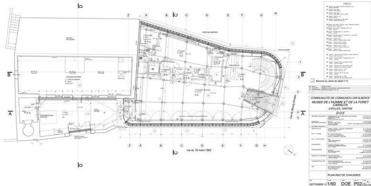
Saboterie et Carnuta : plan des rez-de-chaussée.
