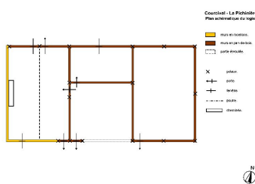
Plan schématique du logis. Dess. Julien Hardy IVR52_20087203084NUDA
