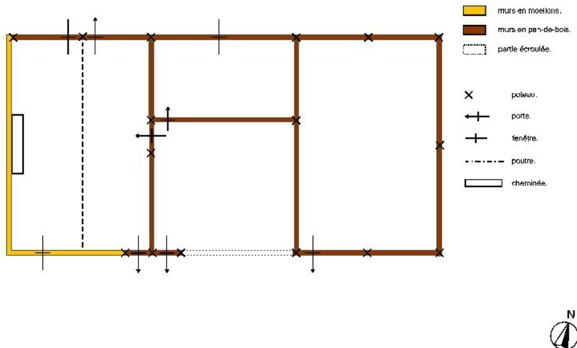
Plan schématique du logis.
