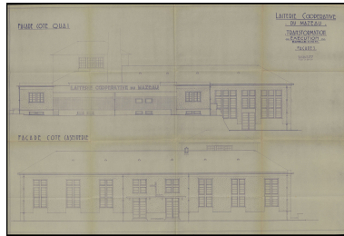
Projet de reconstruction par Gaston Sené, 27 avril 1950 : élévations nord et sud. Repro. Yannis Suire IVR52_20238500294NUCA
