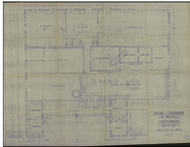
Projet de reconstruction par Gaston Sené, 14 avril 1950 : plan du rez-de-chaussée. Repro. Yannis Suire IVR52_20238500292NUCA
