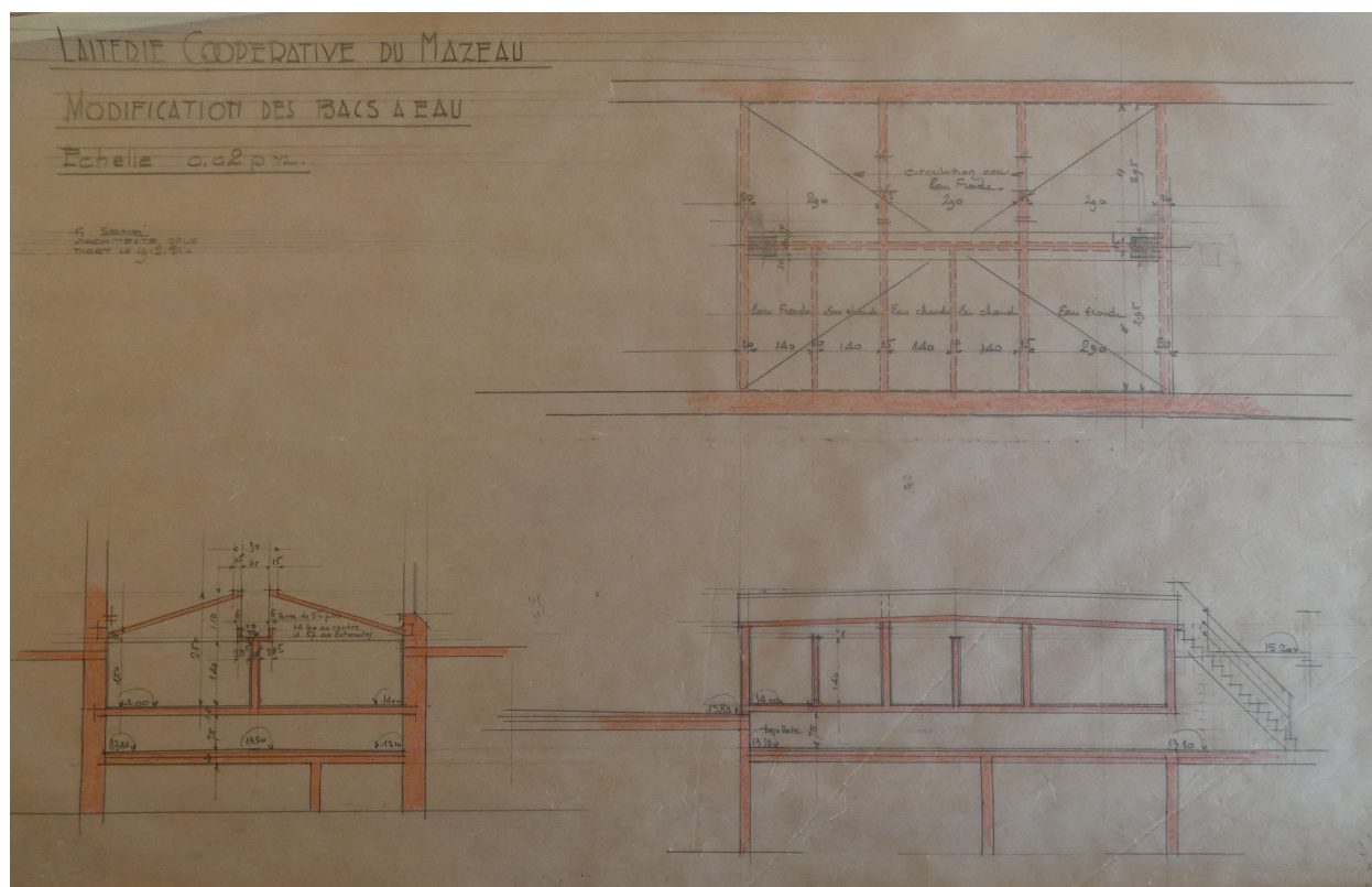
Projet de modification des bacs à eau par Gaston Sené, 19 février 1951.
