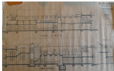
Projet de reconstruction par Gaston Sené, juin 1950 : coupes ouest- est en haut et est-ouest en bas. Repro. Yannis Suire IVR52_20238500299NUCA
