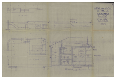
Projet de reconstruction par Gaston Sené, 18 avril 1950 : élévations et plan des réserves à mazout et à charbon. Repro. Yannis Suire IVR52_20238500296NUCA
