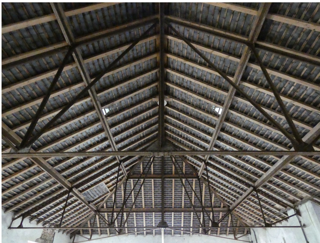
Le grenier à l'étage du corps principal de bâtiment sud, côté ouest : la charpente métallique.
