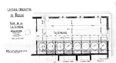
Plan de la caséinerie par Gaston Sené, 16 janvier 1952. Repro. Yannis Suire IVR52_20238500302NUCA
