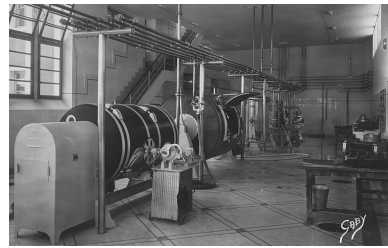
Barattes dans la salle de fabrication du beurre vers 1955. Repro. Yannis Suire IVR52_20238500309NUCA
