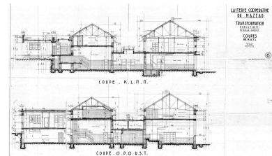
Projet de reconstruction par Gaston Sené, juin 1950 : coupes nord-sud. Repro. Yannis Suire IVR52_20238500303NUCA
