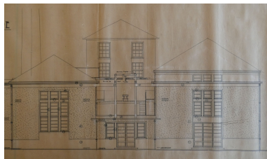
Projet de reconstruction par Gaston Sené, détail de l'élévation ouest avec portique, 26 avril 1950, modifié le 25 octobre 1950. Repro. Yannis Suire IVR52_20238500298NUCA
