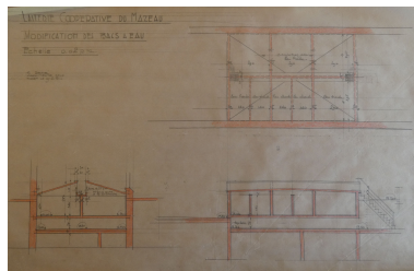
Projet de modification des bacs à eau par Gaston Sené, 19 février 1951. Repro. Yannis Suire IVR52_20238500300NUCA
