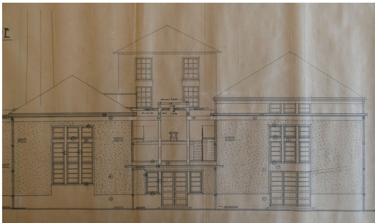
Projet de reconstruction par Gaston Sené, détail de l'élévation ouest avec portique, 26 avril 1950, modifié le 25 octobre 1950.
