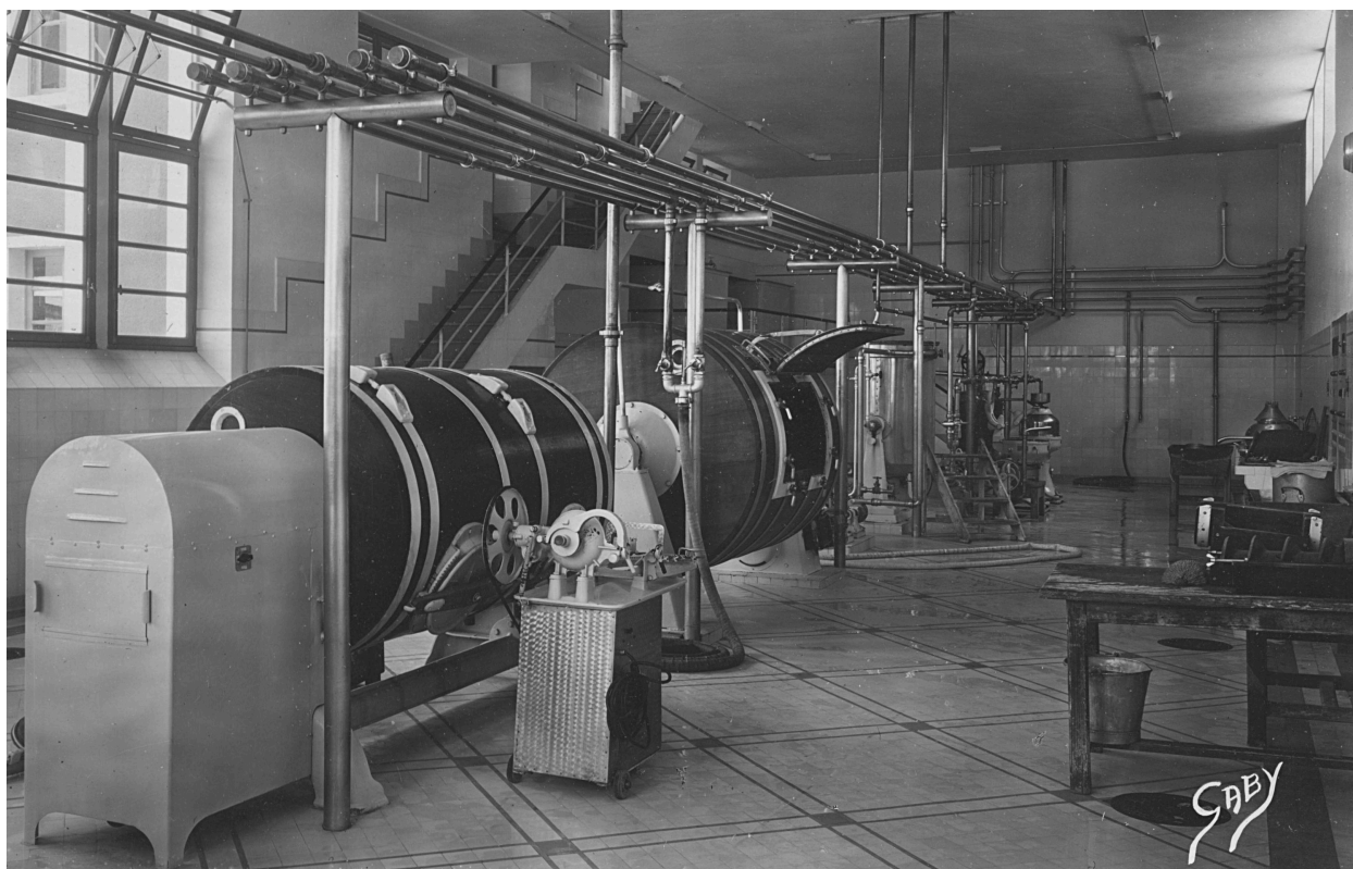
Barattes dans la salle de fabrication du beurre vers 1955.
