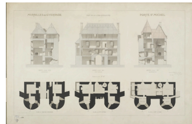
Dessin aquarellé de 1878, coupes et plans. Autr. Emile Boeswillwald, Phot. Denis (reproduction) Pillet IVR52_20064402575NUCA
