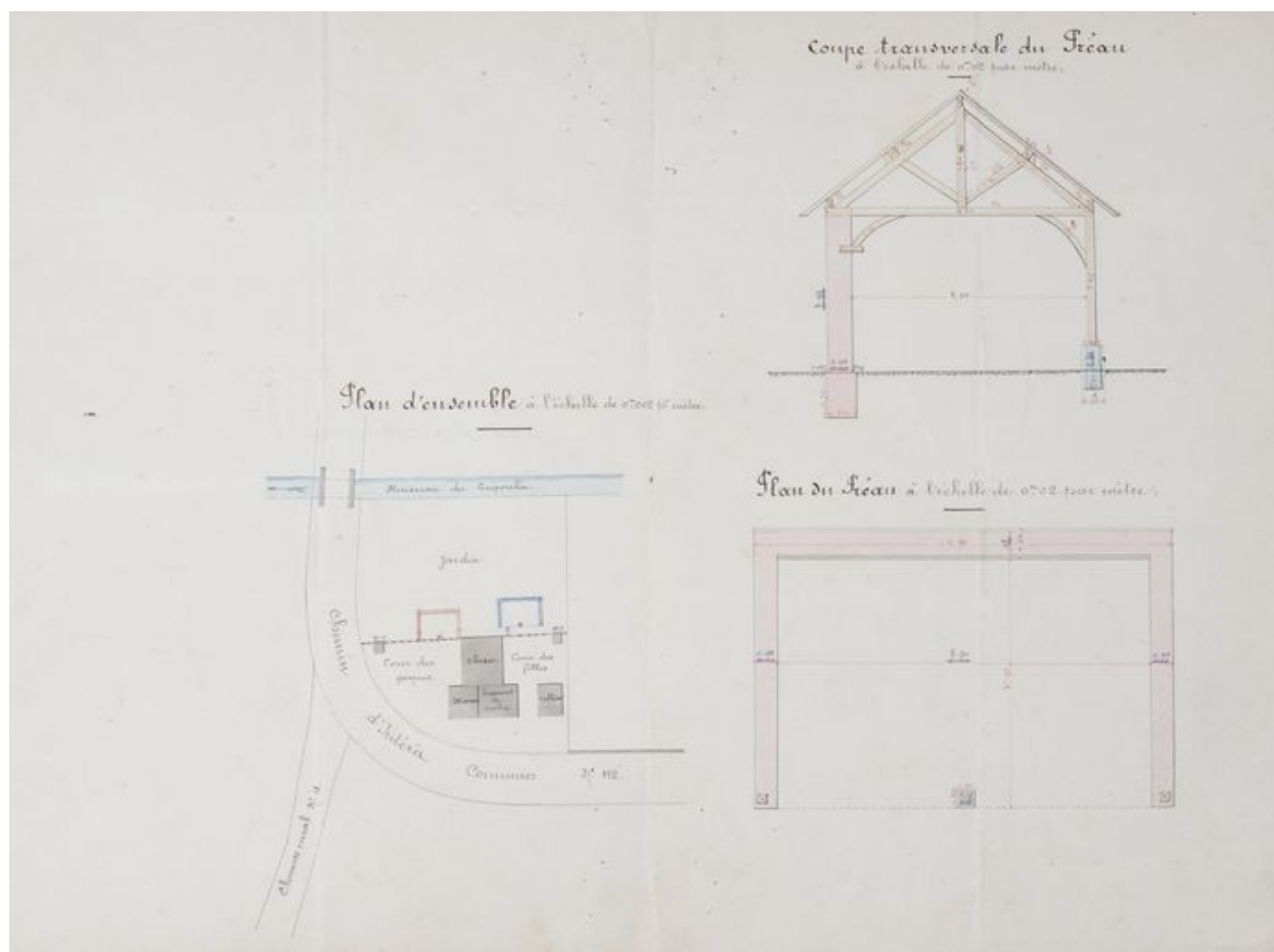
Plan de l'école et plan et coupe du préau à construire. 1910.
