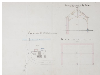
Plan de l'école et plan et coupe du préau à construire. 1910. Autr. Modeste Legendre, Phot. Yves (reproduction) Guillotin IVR52_20107202035NUCA
