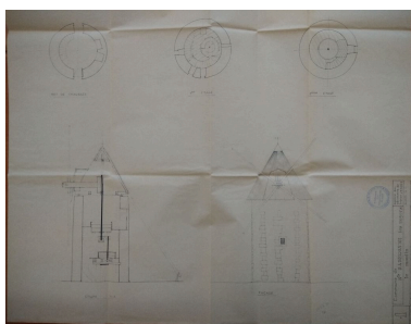
Plan, façade et coupe du moulin en 1978. Phot. Yannis (reproduction) Suire IVR52_20188500998NUC
