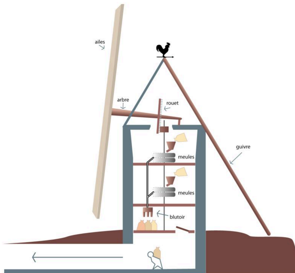
Fonctionnement type d'un moulin à vent
