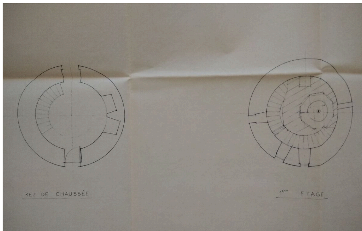
Plan, façade et coupe du moulin en 1978 : plans du rez-de-chaussée et du premier étage.
