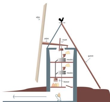
Fonctionnement type d'un moulin à vent. Phot. Jean Jay IVR54_20151709858NUCA
