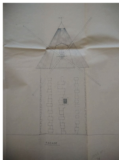
Plan, façade et coupe du moulin en 1978 : élévation. Phot. Yannis (reproduction) Suire IVR52_20188500999NUC
