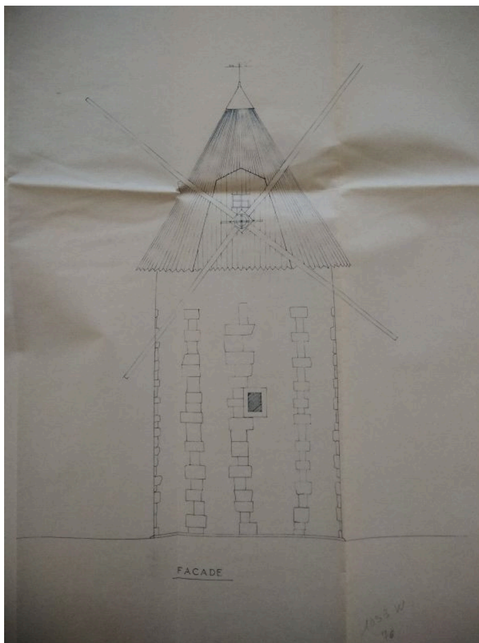
Plan, façade et coupe du moulin en 1978 : élévation.
