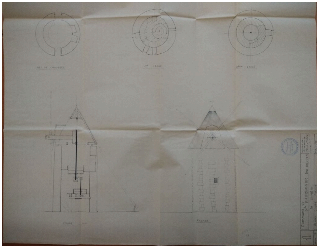
Plan, façade et coupe du moulin en 1978.
