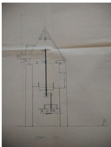
Plan, façade et coupe du moulin en 1978 : coupe. Phot. Yannis (reproduction) Suire IVR52_20188501000NUC
