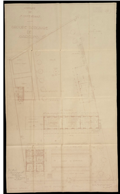
Projet de groupe scolaire de garçons, en 1934 : plan d'ensemble. Autr. René Delamotte, Phot. Bruno Rousseau, Phot. Youenn (reproduction) Communeau IVR52_20124901260NUCA
