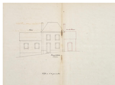
Mairie-école de Montreuil-le-Henri : plan en élévation, 1874. Repro. Pierre-Bernard Fourny IVR52_20267200026NUCA
