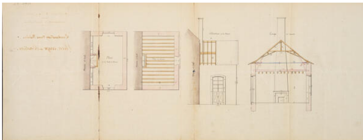
Mairie-école de Montreuil-le-Henri : plan au sol, coupe et élévation, 1874.
