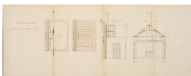
Mairie-école de Montreuil-le-Henri : plan au sol, coupe et élévation, 1874. Repro. Pierre-Bernard Fourny IVR52_20267200028NUCA
