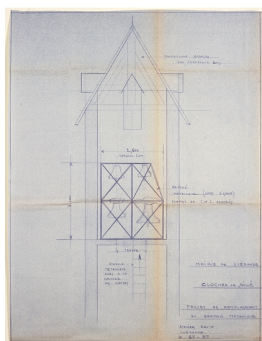
Projet de remplacement du beffroi métallique. Dressé par Atelier David, 1959. Phot. Denis (reproduction) Pillet IVR52_20084400407NUCA
