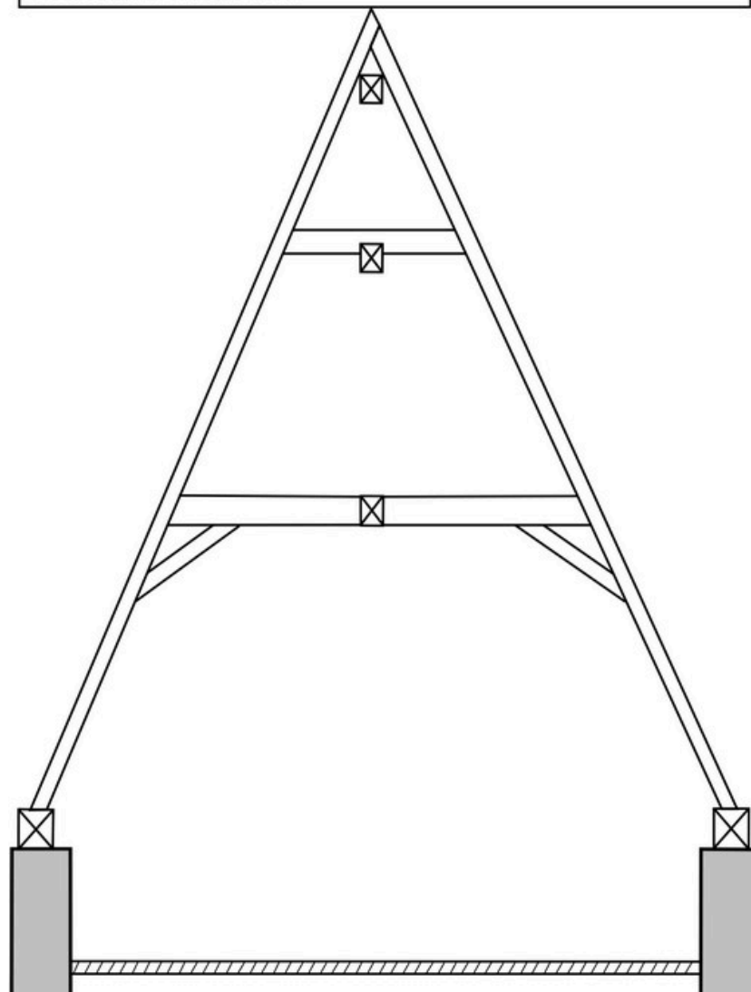
Charpente du pavillon du logis : élévation schématique d'une ferme secondaire.
