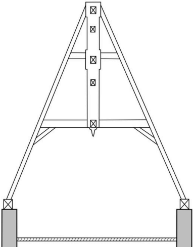
Charpente du pavillon du logis : élévation schématique de la ferme principale ouest. Dess. Nicolas Foisneau IVR52_20095300597NUD
