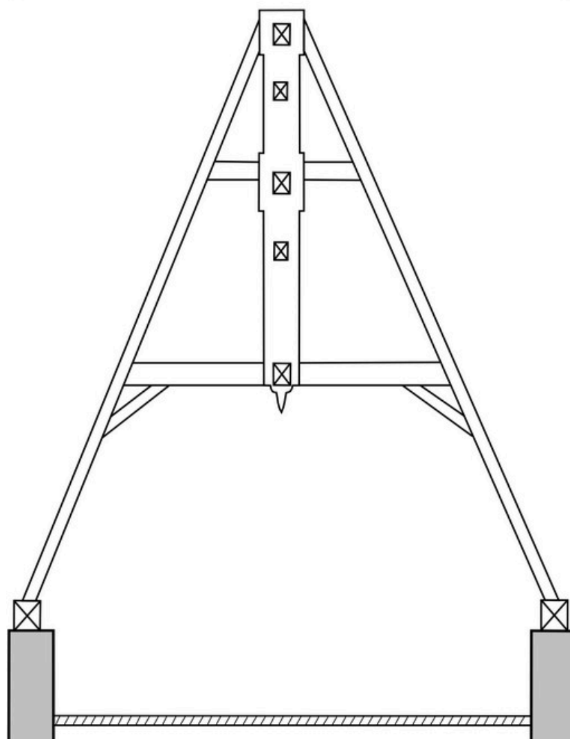
Charpente du pavillon du logis : élévation schématique de la ferme principale ouest.
