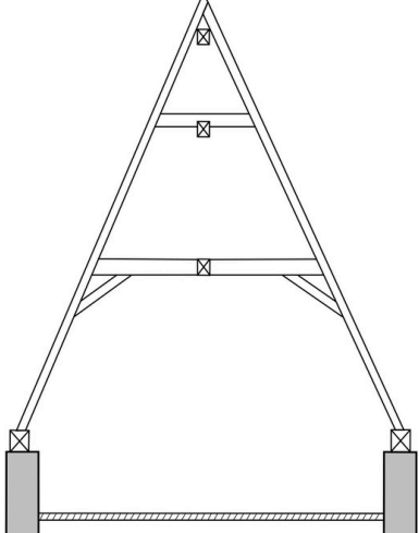
Charpente du pavillon du logis : élévation schématique d'une ferme secondaire. Dess. Nicolas Foisneau IVR52_20095300598NUD
