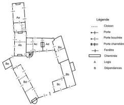
Plan schématique du rez-de-chaussée du manoir et de ses dépendances. Dess. Nicolas Foisneau IVR52_20095300596NUD
