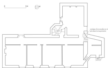
Plan schématique de l'étage, d'après A. Sébilo 2000. (Dessin, V. Desvigne, 2010). Autr. Aurélia Sébilo, Dess. Virginie Desvigne IVR52_20104400557NUDA
