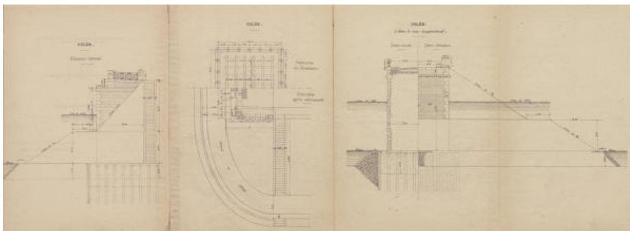
Consolidation du pont de Thouaré. Plan et élévation des culées, 1924.
