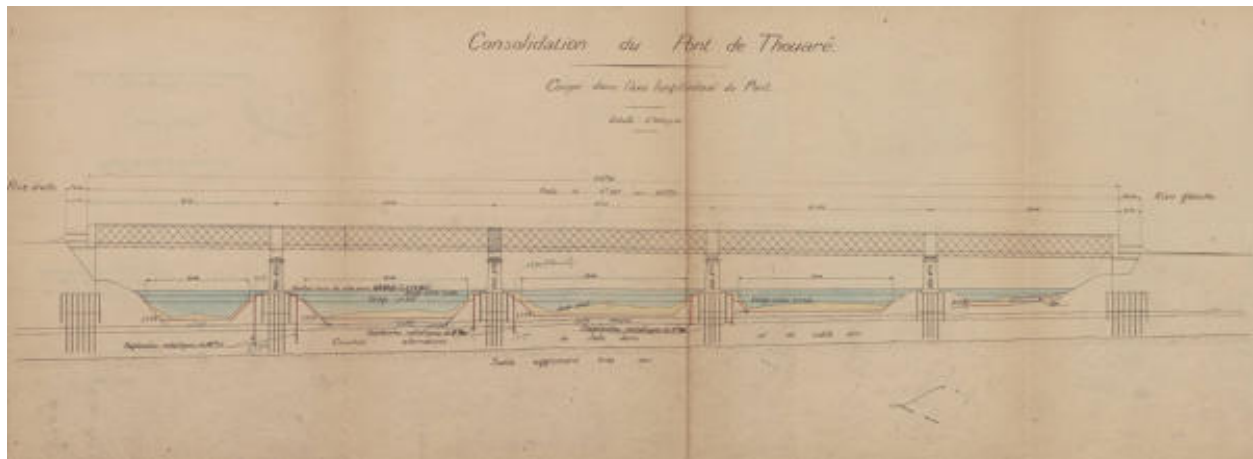
Consolidation du pont de Thouaré. Coupe longitudinale dans l'axe du pont, 1924.
