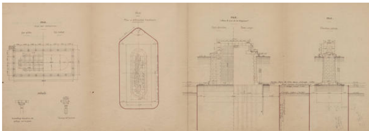
Consolidation du pont de Thouaré. Plan et élévation des piles, 1924.
