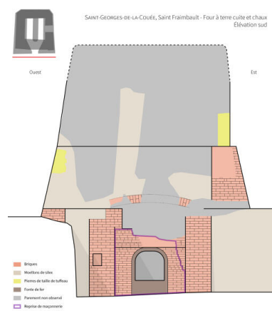
Le four : relevé de l'élévation. Dess. Théo Ben Makhad IVR52_20257200719NUDA
