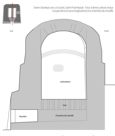
Le four : coupe longitudinale. Dess. Théo Ben Makhad IVR52_20257200717NUDA
