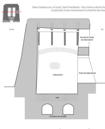
Le four : coupe transversale. Dess. Théo Ben Makhad IVR52_20257200718NUDA
