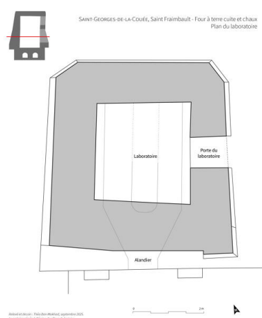
Le four : relevé en plan. Dess. Théo Ben Makhad IVR52_20257200716NUDA
