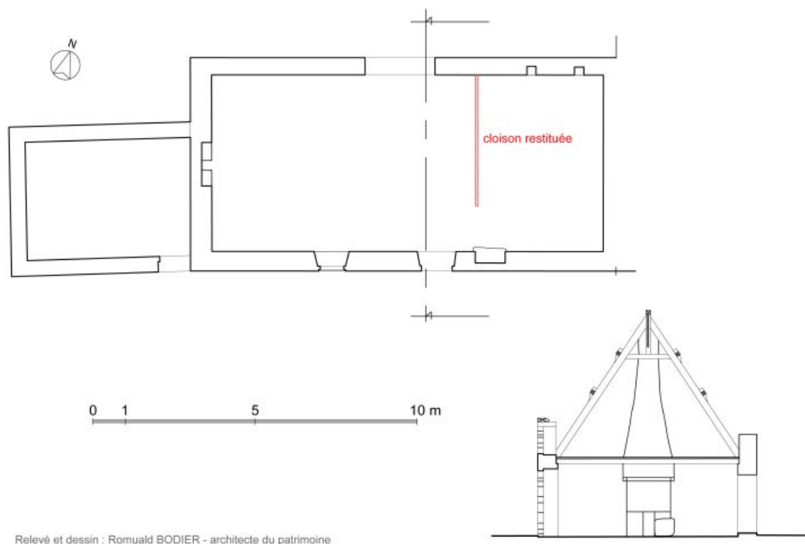
Plan et coupe du premier logis. Dessin R. Bodier, 2009.
