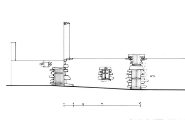
Elévation du premier logis. Dessin R. Bodier, 2009. Dess. Romuald Bodier IVR52_20104400899NUDA
