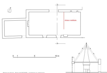
Plan et coupe du premier logis. Dessin R. Bodier, 2009. Dess. Romuald Bodier IVR52_20104400900NUDA
