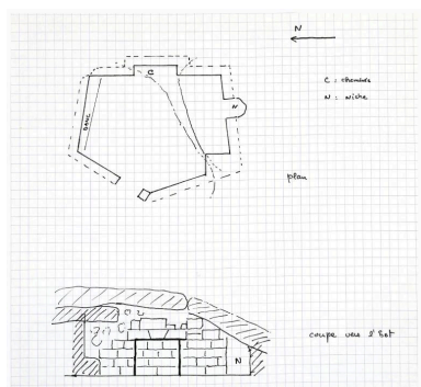
Plan et coupe schématiques, établis lors du pré-inventaire de 1979. Phot. Bruno (reproduction) Rousseau, Phot. Youenn (reproduction) Communeau IVR52_20104902199NUCA
