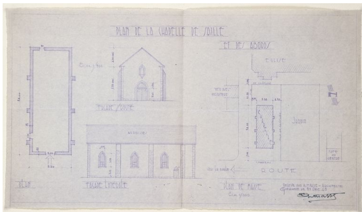
Plan de la chapelle Notre-Dame-de-la-Salette. Dressé par A. Massé, architecte, 1948.
