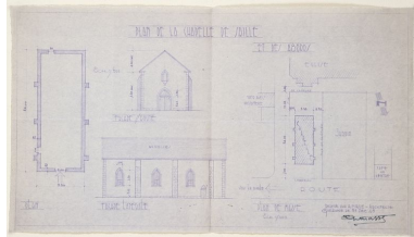
Plan de la chapelle Notre-Dame-de-la-Salette. Dressé par A. Massé, architecte, 1948. Autr. Auguste Macé, Phot. Denis (reproduction) Pillet IVR52_20084402565NUCA
