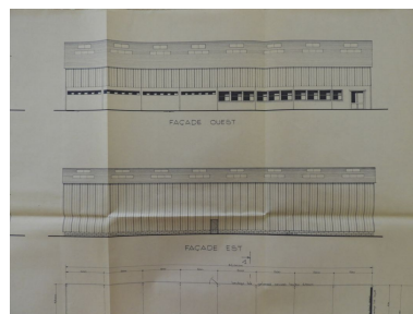
Projet d'atelier pour le chantier naval Pouvreau, 16 mars 1972 : élévation ouest et est. Phot. Yannis (reproduction) Suire IVR52_20198503664NUCA
