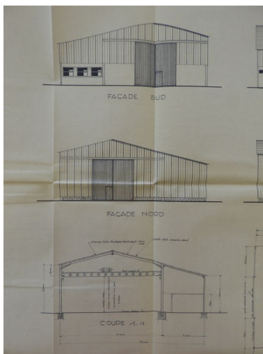
Projet d'atelier pour le chantier naval Pouvreau, 16 mars 1972 : élévations nord et sud, coupe. Phot. Yannis (reproduction) Suire IVR52_20198503663NUCA
