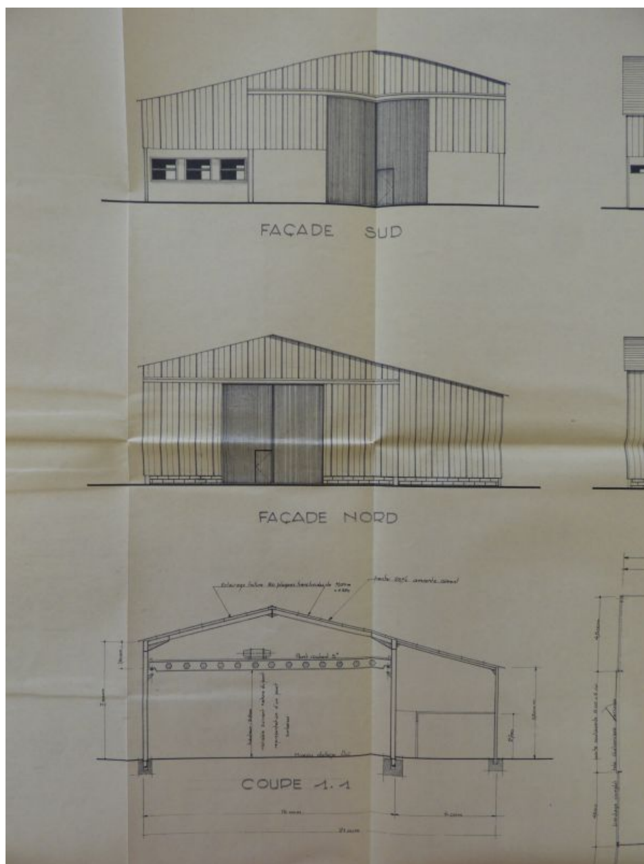
Projet d'atelier pour le chantier naval Pouvreau, 16 mars 1972 : élévations nord et sud, coupe.
