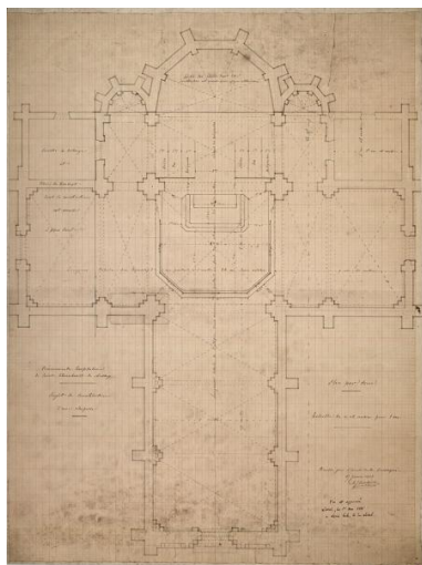
Plan et élévations pour la construction de la chapelle du Sacré-Coeur, communauté hospitalière Saint- Fraimbault, Vendrion, 1888. Repro. Morgane Acou-Le Noan IVR52_20205300455NUCA
