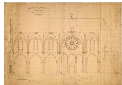
Plan et élévations pour la construction de la chapelle du Sacré-Coeur, communauté hospitalière Saint- Fraimbault, Vendrion, 1888. Repro. Morgane Acou-Le Noan IVR52_20205300456NUCA
