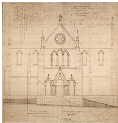
Plan et élévations pour la construction de la chapelle du Sacré-Coeur, communauté hospitalière Saint- Fraimbault, Vendrion, 1888. Repro. Morgane Acou-Le Noan IVR52_20205300453NUCA
