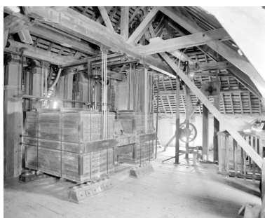
Comble du moulin. Le plansichter. Phot. François Lasa IVR52_20015300602X
