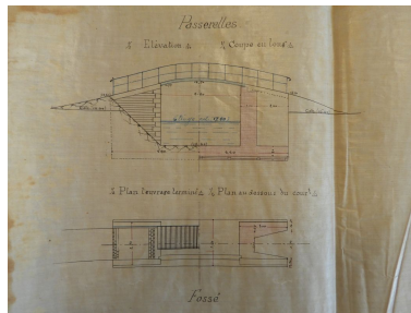
Projet de passerelles aux extrémités du canal à creuser dans les marais de Charouin, 9 novembre 1892 : élévation, plan et coupe. Phot. Yannis (reproduction) Suire IVR52_20198503668NUCA
