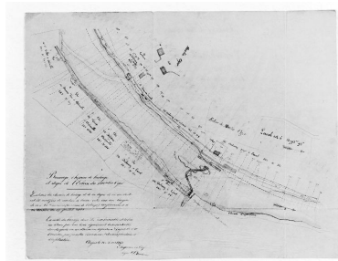
Plan d'ensemble du site : anciens barrage et moulin (détruits, à l'exception de la maison du meunier), nouveau barrage à écluse (réalisé). Autr. Charles Dupuy, Repro. François Lasa
