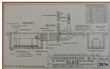
Plan type d'une fosse à essence de la société l'Economique, pour la station de Louis Germond, à Maillé, 1931. Phot. Yannis (reproduction) Suire IVR52_20218501502NUCA
