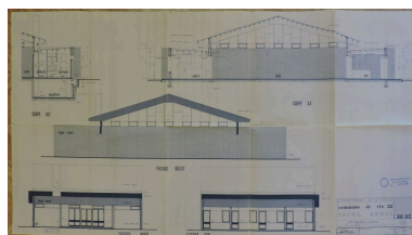
Projet de foyer rural, par Guy Durand, 1970 : élévations et coupes.
