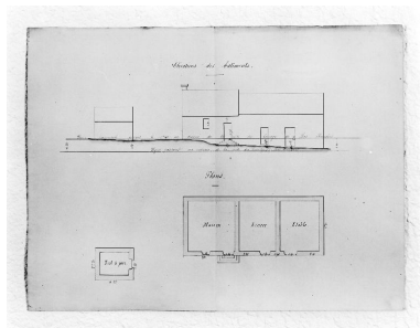
Plan et élévation des anciennes dépendances du moulin d'Hambert, actuellement maison du Port.
