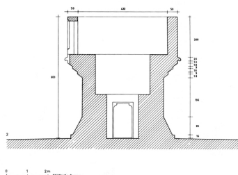
Moulin de Crémeur. Relevé en coupe du moulin. 1972. Autr. Jean-Claude Delesne, Phot. Christian (reproduction) Cussonneau IVR52_20094401466NUCA
