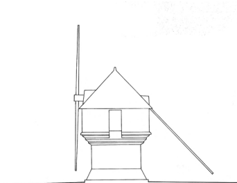
Moulin de Crémeur. Élévation schématique du moulin. 2009. Reprise de fond. Autr. Jean-Claude Delesne, Phot. Christian (reproduction) Cussonneau IVR52_20094401465NUCA
