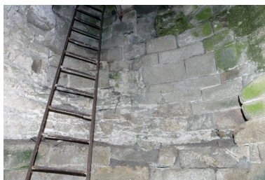
Vue intérieure du pied ; détail des buchages à l'emplacement du petit escalier primitivement accessible par une échelle et permettant d'atteindre l'étage. Phot. Denis Pillet IVR52_20074401523NUCA
