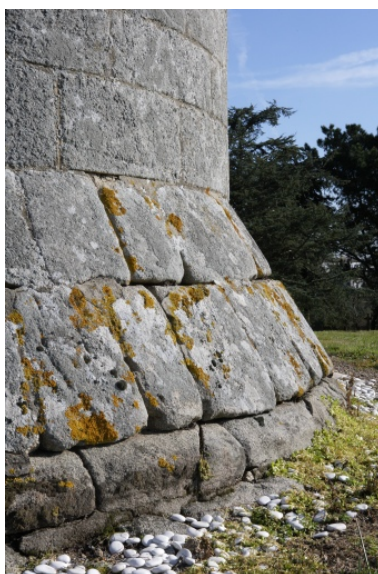
Pied de la tour. Détail de l'empattement. Phot. Denis Pillet IVR52_20074401520NUCA
