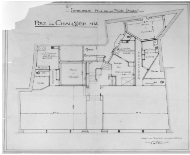
Plan du rez-de-chaussée n° 2, par H. Palausi, 1914. Repro. François Lasa, Autr. Henri Palausi IVR52_19924900474X
