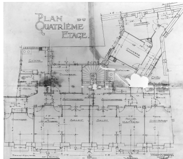
Plan du 4e étage, par H. Palausi, 1914. Repro. François Lasa, Autr. Henri Palausi IVR52_19924900865V
