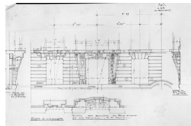
Façade antérieure, partie gauche, entresol : détail d'élévation plan et coupes, par H. Palausi, 1914. Repro. François Lasa, Autr. Henri Palausi IVR52_19924900477X
