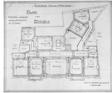
Plan des étages, avec un seul appartement par niveau, relevé portant la mention annulé, par H. Palausi, 1914. Repro. François Lasa, Autr. Henri Palausi IVR52_19924900475X
