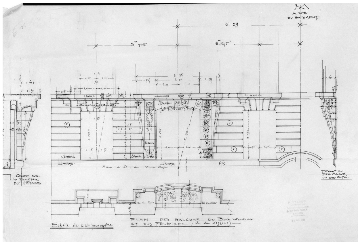
Façade antérieure, partie gauche, entresol : détail d'élévation plan et coupes, par H. Palausi, 1914.
