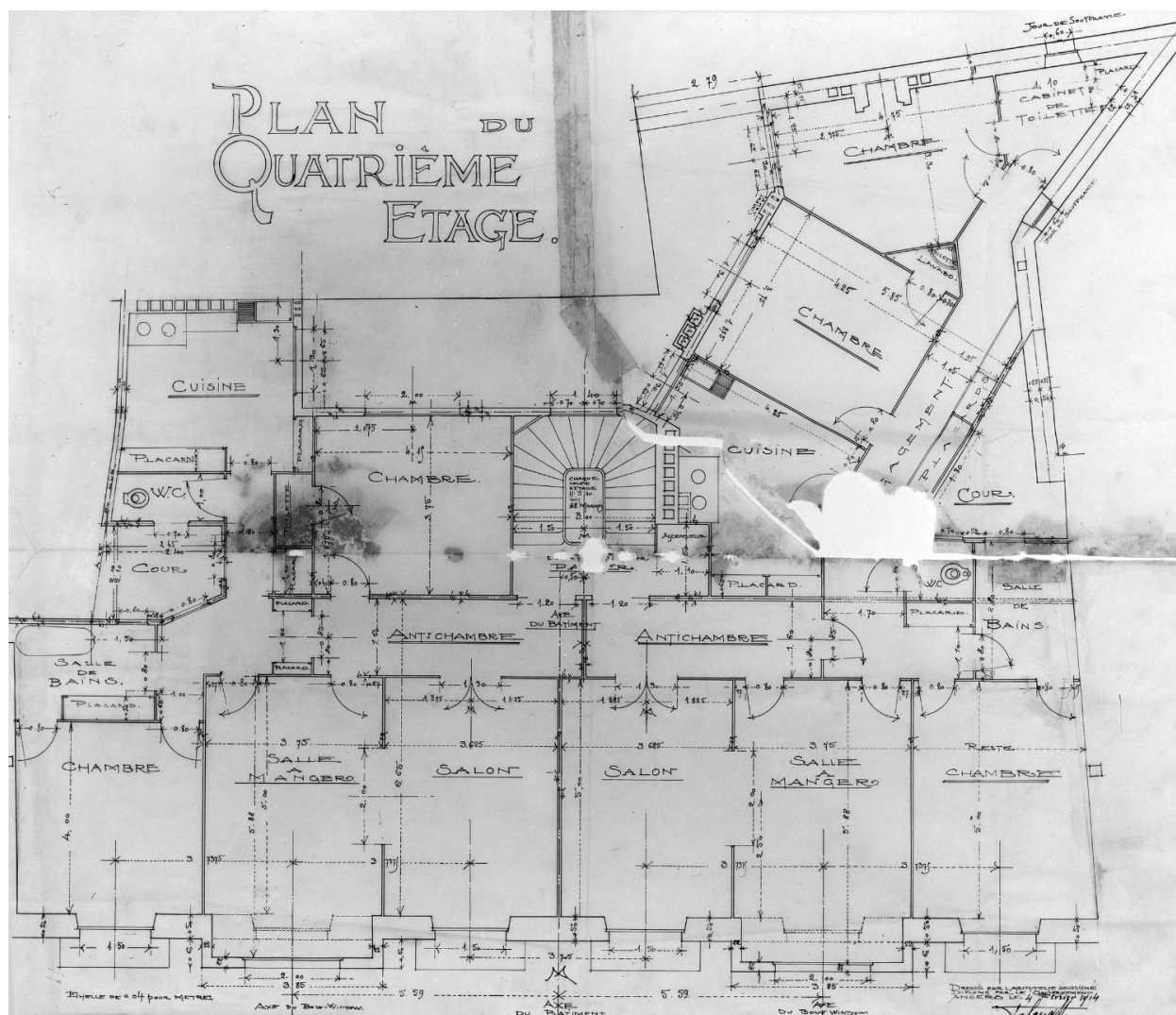
Plan du 4e étage, par H. Palausi, 1914.
