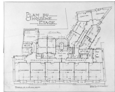
Plan du 5e étage, par H. Palausi, 1914. Repro. François Lasa, Autr. Henri Palausi IVR52_19924900472X
