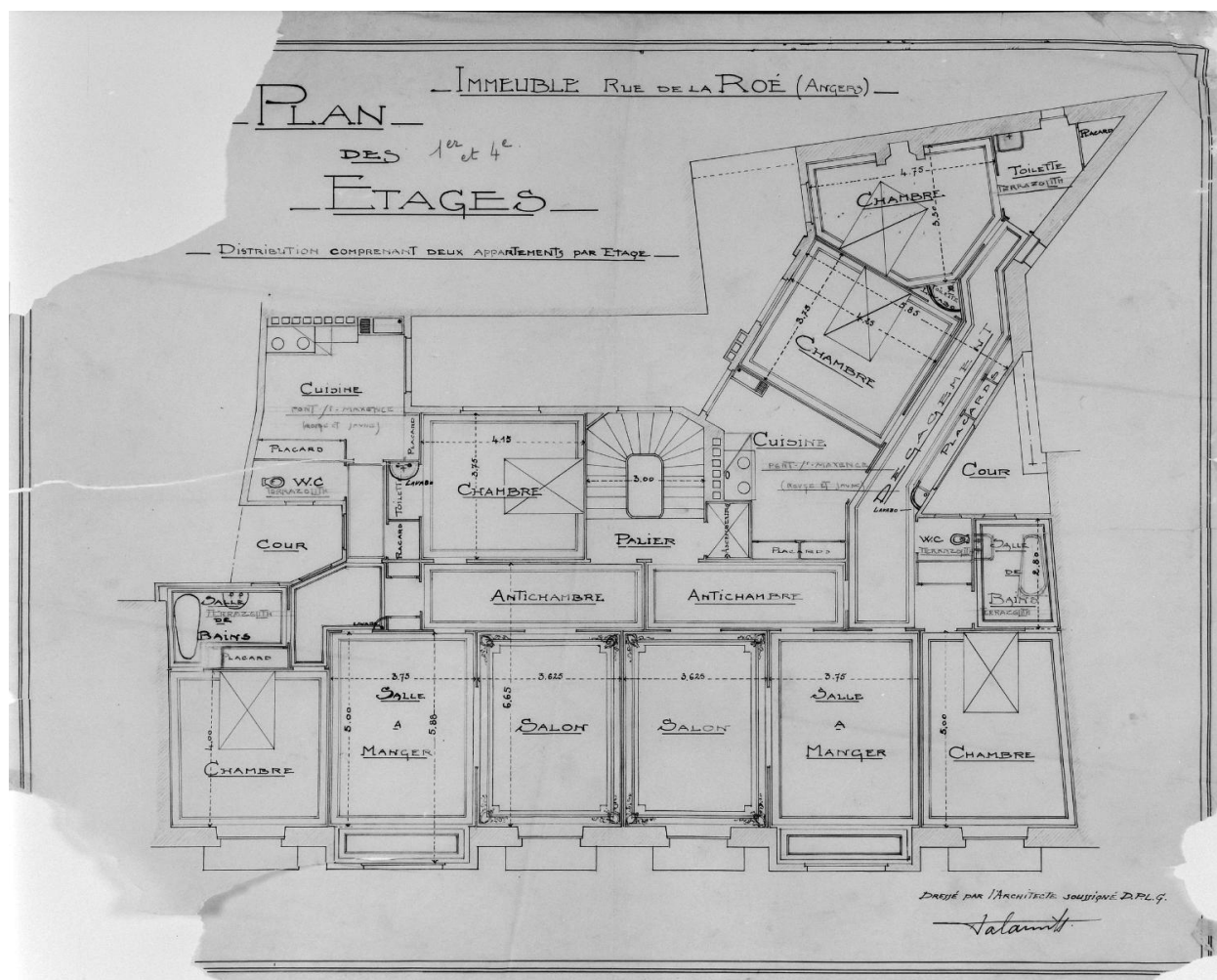
Plan des étages : 1er et 4e projets avec deux appartements par niveaux, par H. Palausi, 1914.
