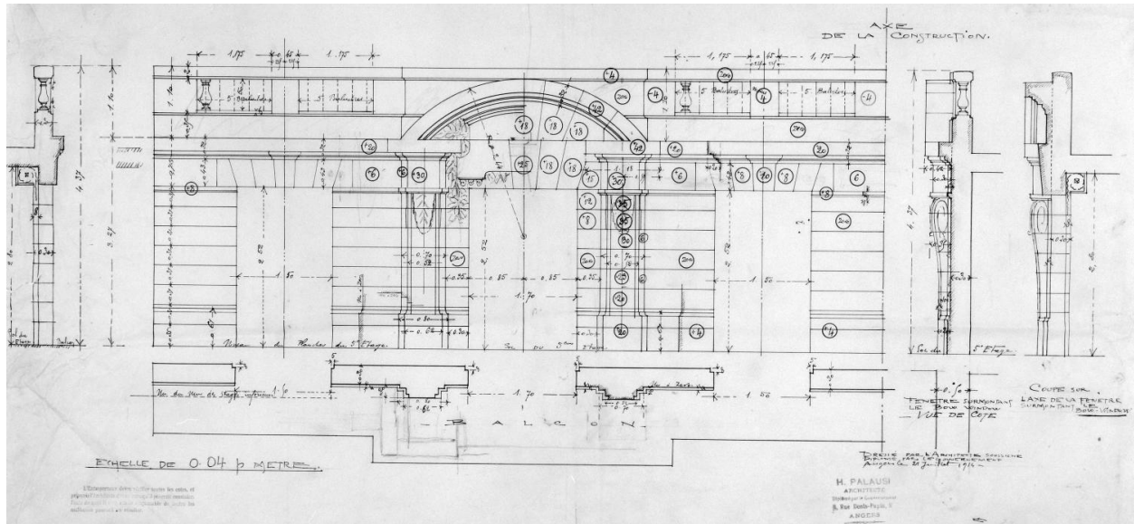
Façade antérieure, étage attique, partie gauche : détail d'élévation, par H. Palausi, 1914.
