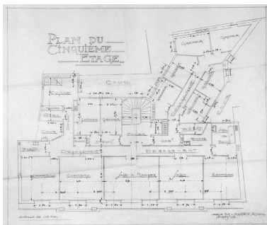
Plan du 5e étage, par H. Palausi, 1914. Repro. François Lasa, Autr. Henri Palausi IVR52_19924900473X
