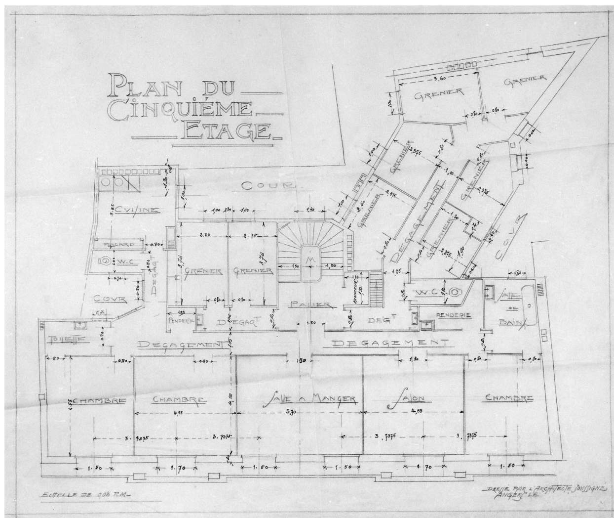
Plan du 5e étage, par H. Palausi, 1914.
