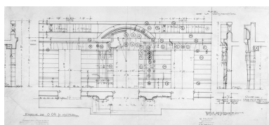
Façade antérieure, étage attique, partie gauche : détail d'élévation, par H. Palausi, 1914. Repro. François Lasa, Autr. Henri Palausi IVR52_19924900478X
