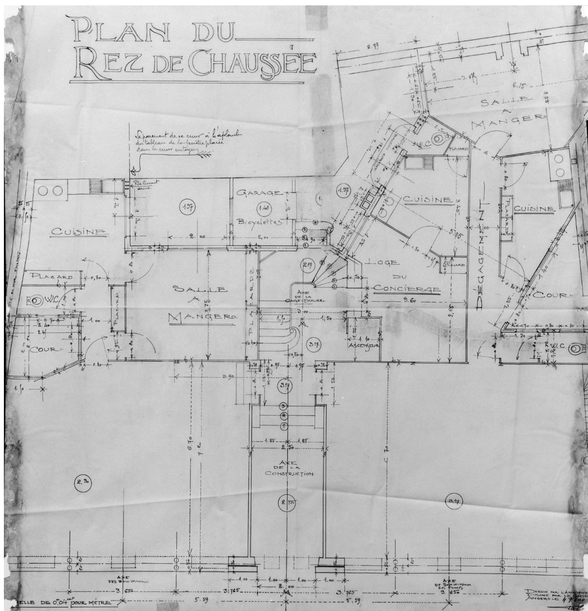
Plan du rez-de-chaussée, par H. Palausi, 1914.
