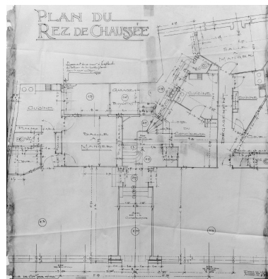
Plan du rez-de-chaussée, par H. Palausi, 1914. Repro. François Lasa, Autr. Henri Palausi IVR52_19924900471X
