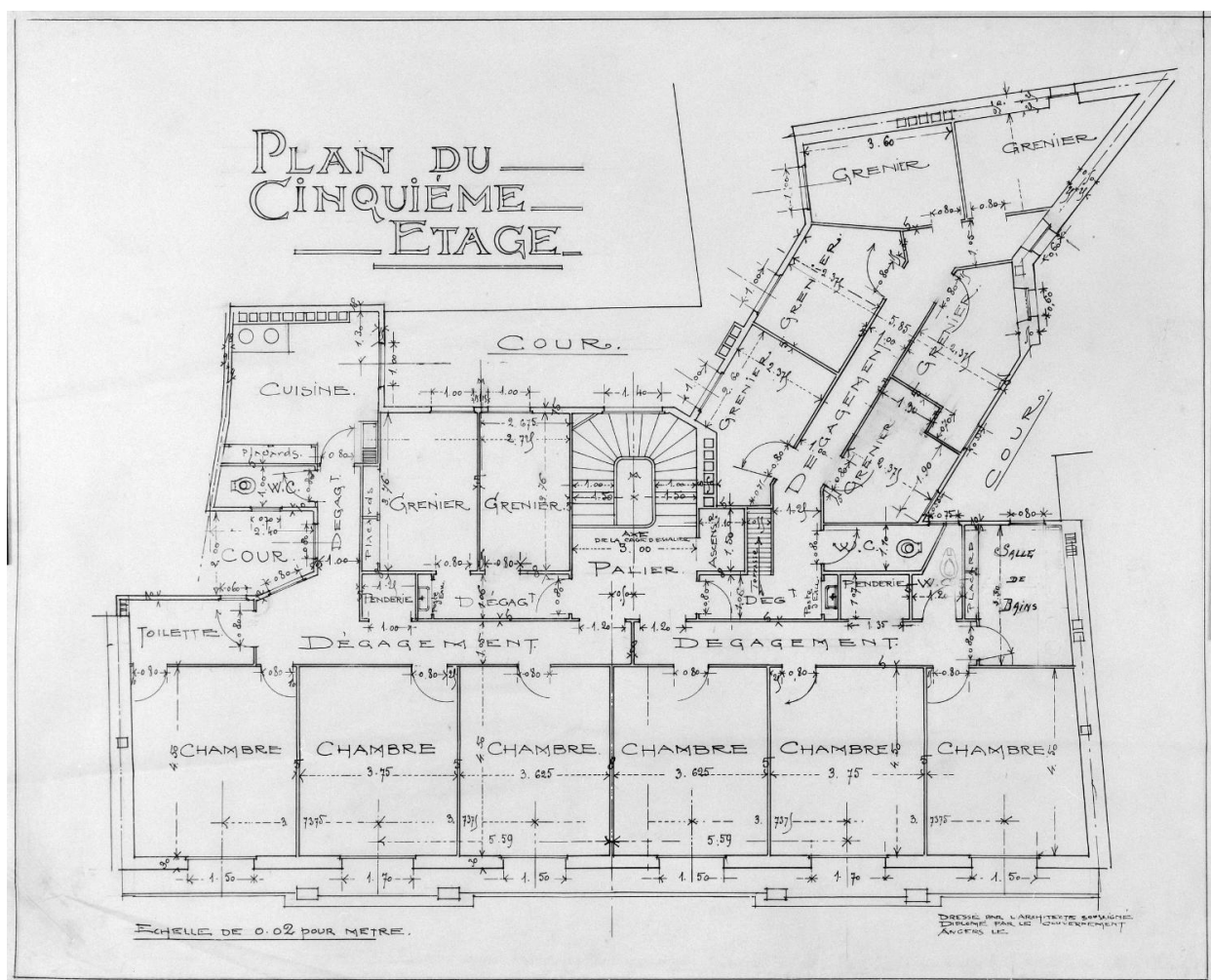
Plan du 5e étage, par H. Palausi, 1914.
