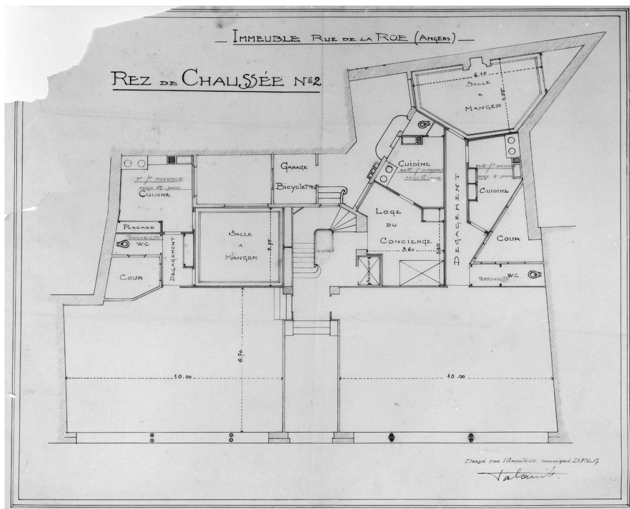
Plan du rez-de-chaussée n° 2, par H. Palausi, 1914.
